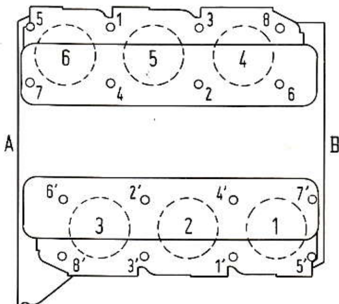
Schema dell'ordine di serraggio delle viti di fissaggio delle teste al gruppo cilindri.
