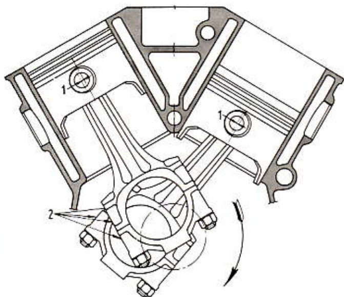
Schema per il montaggio del gruppo biella-stantuffo nei cilindri.
