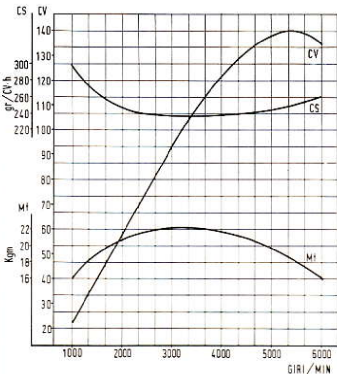
Curve caratteristiche del motore, rilevate con il metodo DIN.
